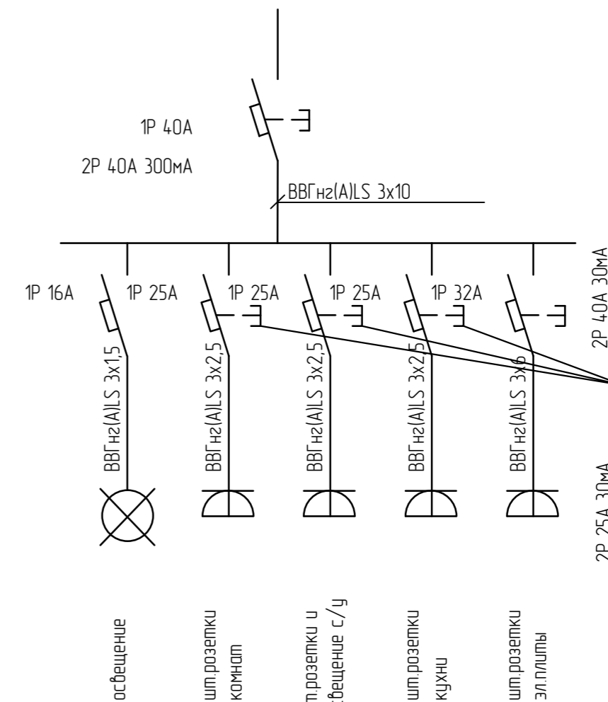
Принципиальная схема квартирного щитка
