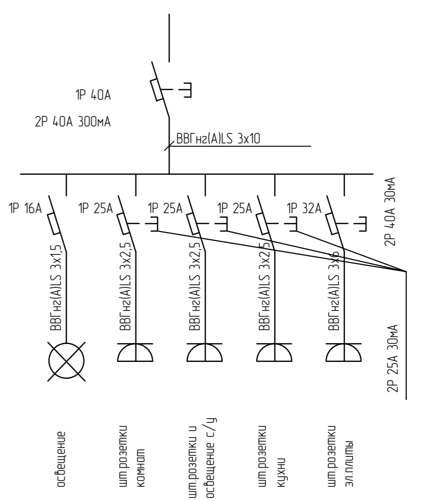
Принципиальная схема квартирного щитка
